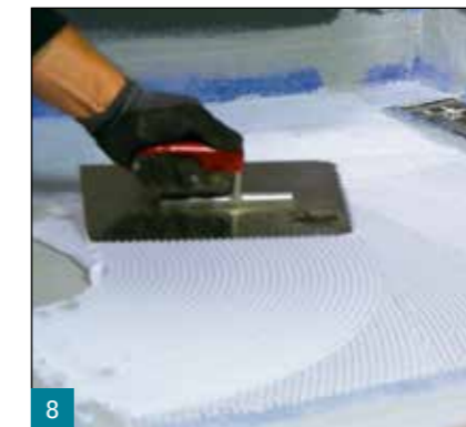
8 Die erste Lage mit einem 4 mm Zahnglätter aufkämmen und anschließend glätten.
