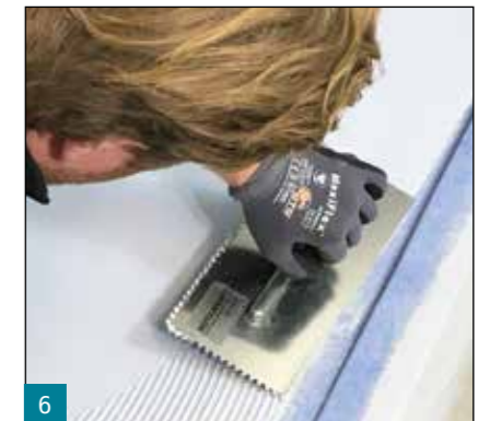
6 Bei den Wassereinflussklassen W2-I und W3-I sowie auf Balkonen und Terrassen wird MULTIPROOF® in einer Mindesttrockenschichtdicke von 2,0 mm aufgetragen.
