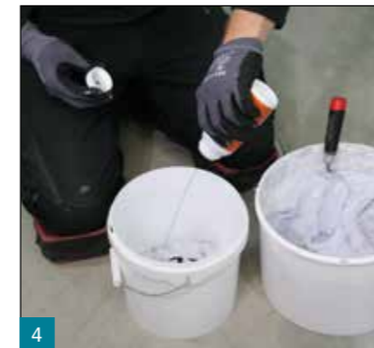
4 Zur Herstellung der Kontrastfarbe (bei der Verwendung von MULTIPROOF® als Dichtfolie) wird für die zweite Lage DF Color Farbpigment hinzugegeben.
